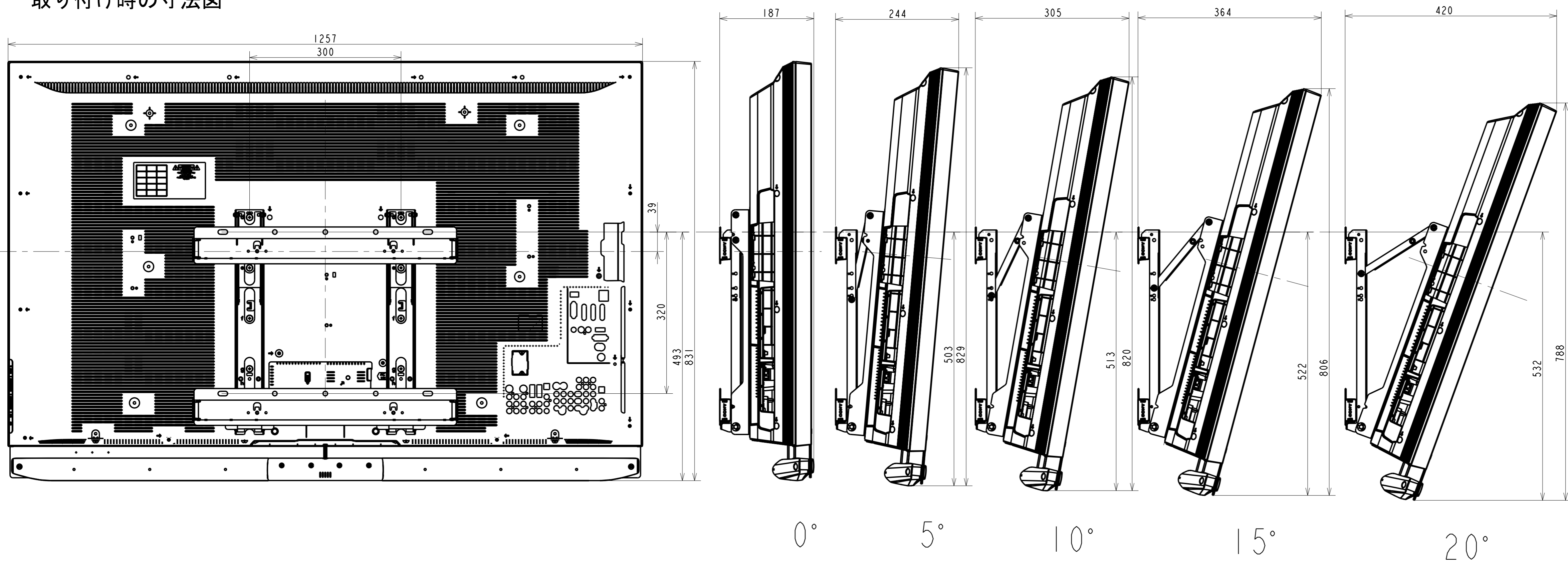
壁掛けユニット 取り付け時の寸法図
