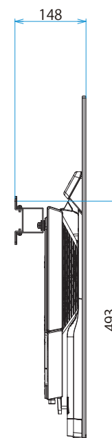
標準壁掛け (SU-WL450)
